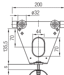
Mitnehmerwagen
