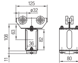
Mitnehmerwagen
