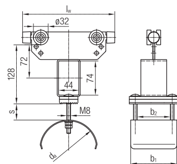
Mitnehmerwagen
