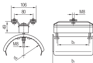
Endklemme
