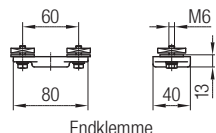
Endklemme
