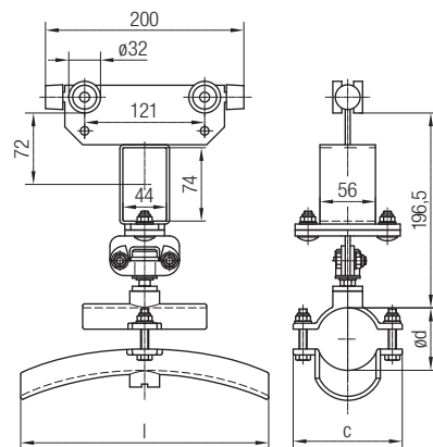
Mitnehmerwagen
