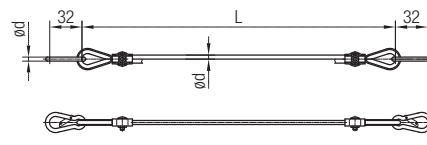
Ausführung B (mit Karabinerhaken)
