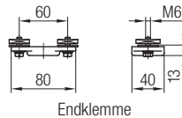
Endklemme
