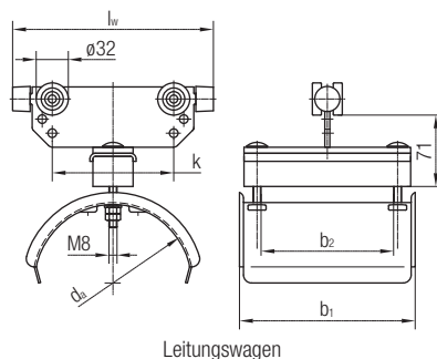
Leitungswagen
