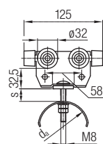
Leitungswagen
