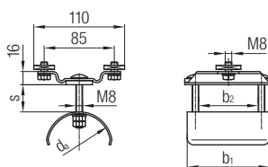
Endklemme
