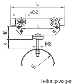
Leitungswagen
