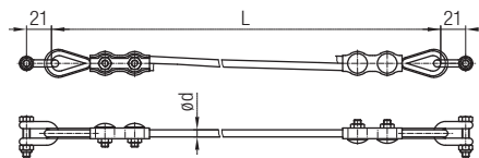
Ausführung A (Schäkel)
