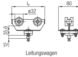
Leitungswagen
