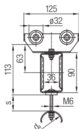
Mitnehmerwagen
