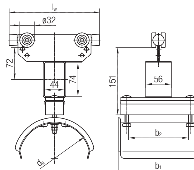
Mitnehmerwagen
